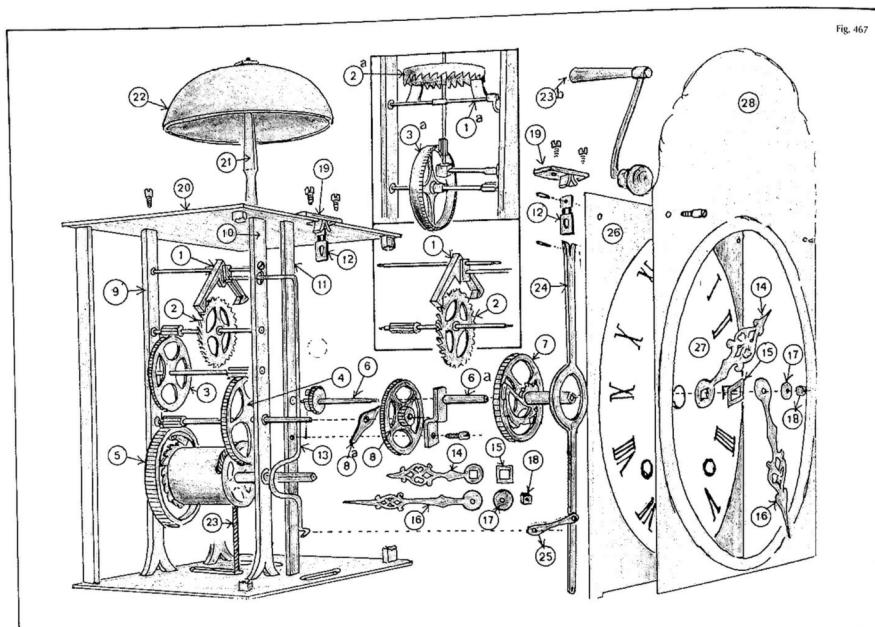
Fig. 467. Le mécanisme d'une comtoise, côté mouvement.
